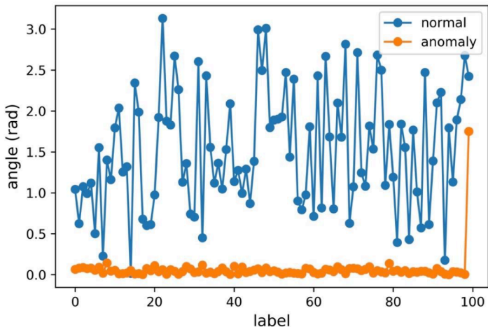
基于角度的异常检测案例
