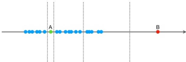
IForest 一维示例
