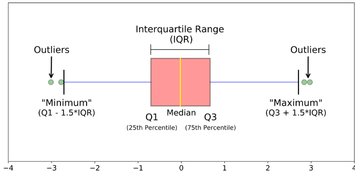
Boxplot 中的异常值区分
